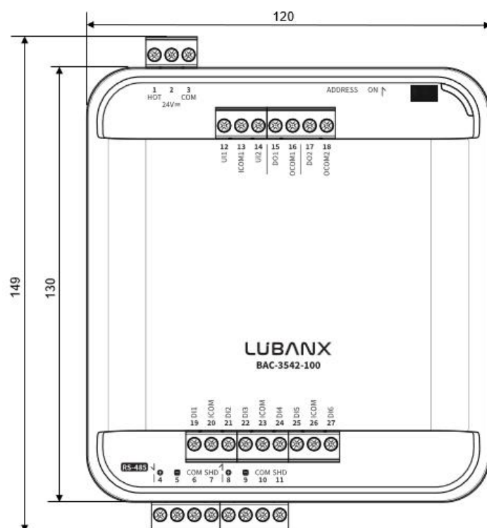
正面尺寸(单位: mm)
