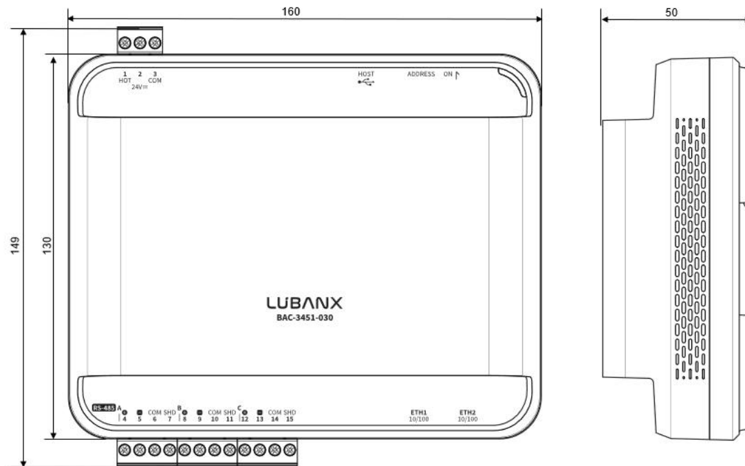
正面尺寸(单位: mm)
