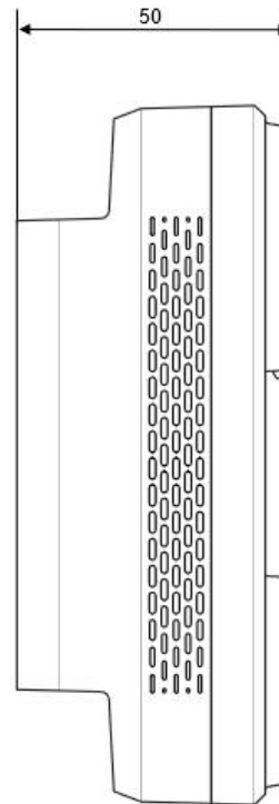
侧面尺寸(单位: mm)
