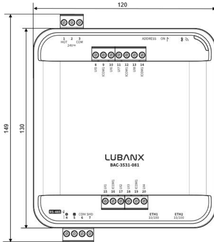
正面尺寸(单位: mm)
